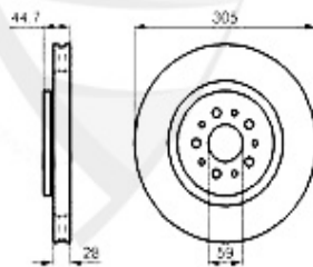
4. BS 101651 3.0/3.2 V6 24V vorne/front
