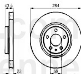
3. BS 518751 V6 12V/ 2.0 V6 Turbo vorne/front
