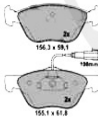
4. 21636 V6 12V #06009487> vorne/front
