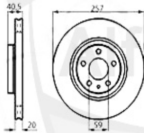
4. BS 101651 3.0/3.2 V6 24V vorne/front
