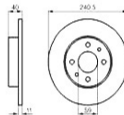
5. BS 516711 hinten/rear
