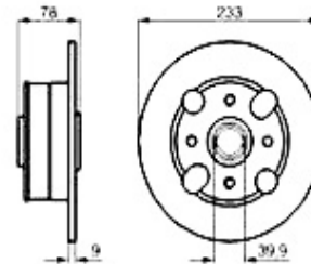
5. BS 100615 hinten/rear
