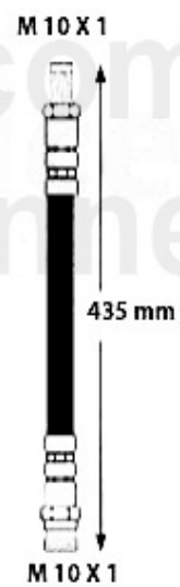
3. BS 511666 hinten/rear
