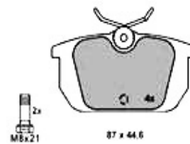
6. 21103 hinten/rear
