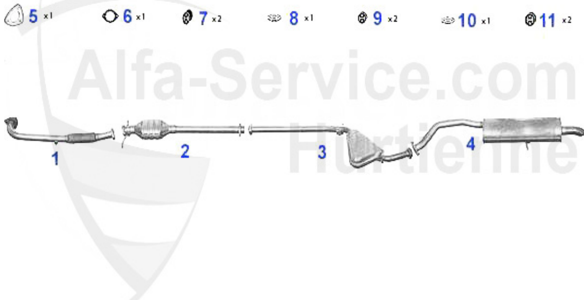
166 2.4 JTD TURBO DIESEL 20V
