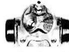
2. RBZ 178 rechts/right System: Bendix Ø 17,46 mm > 1986 - 4x4
